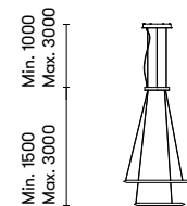
N Ø900 mm 76W Ø600 mm 7296 lm
