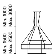
J Ø600 mm 207W Ø1200 mm 17280 lm Ø1200 mm Ø600 mm
