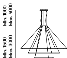
G Ø3000 mm 368W Ø2000 mm 30720 lm Ø1200 mm
